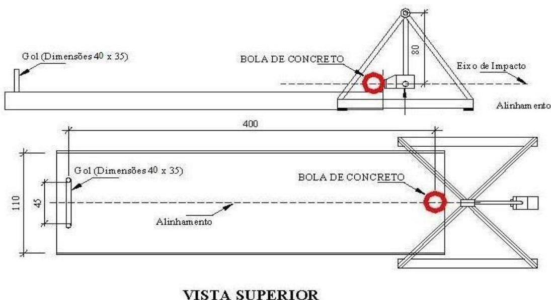
Figura 1 – Equipamento de impulso, pista de rolamento e gol.
